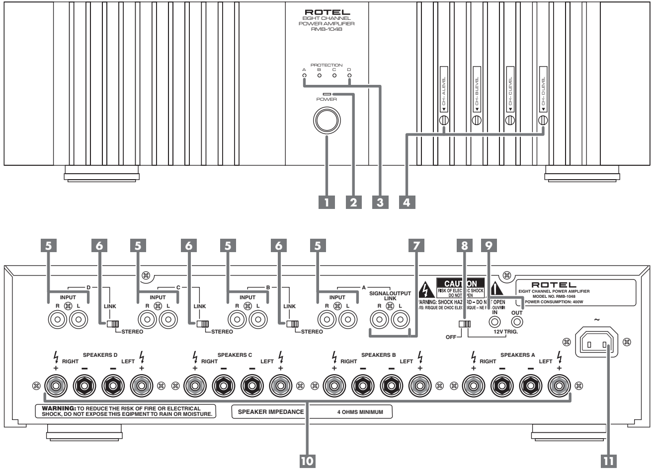
Figure 1: Controls and Connections Commandes et branchements Bedienelemente und Anschlüsse Controlli e Collegamenti Controlos y Conexiones Bedieningsorganen en aansluitingen Funktioner och anslutningar
